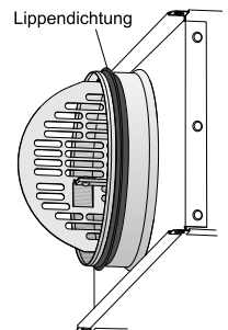
Anschlussstutzen mit Lippendichtung
